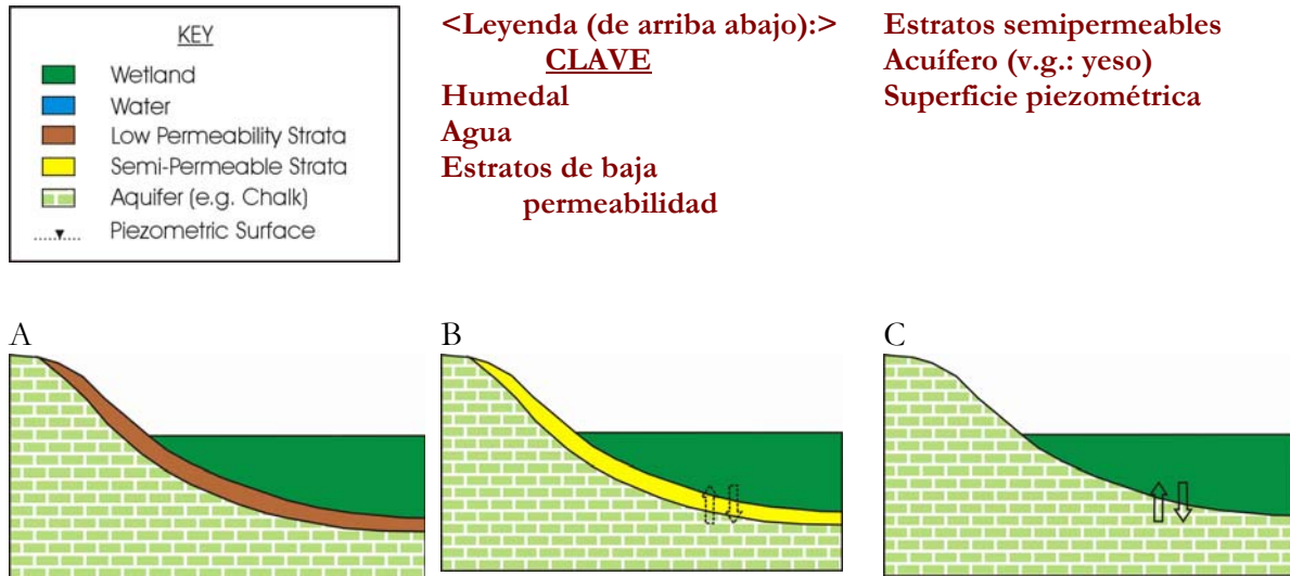
Figura 2. Diferentes tipos de acuíferos. a) acuífero y humedal separados por rocas impermeables (acuícludo): no hay interacción; b) acuífero y humedal separados por rocas de baja permeabilidad (acuitardo): escasa interacción; y c) acuífero y humedal separados por rocas de elevada permeabilidad o no separados: fuerte interacción (véase la figura 3 a propósito de la clave).
